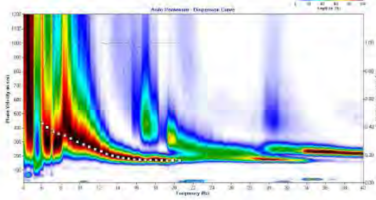
CURVA DI DISPERSIONE
