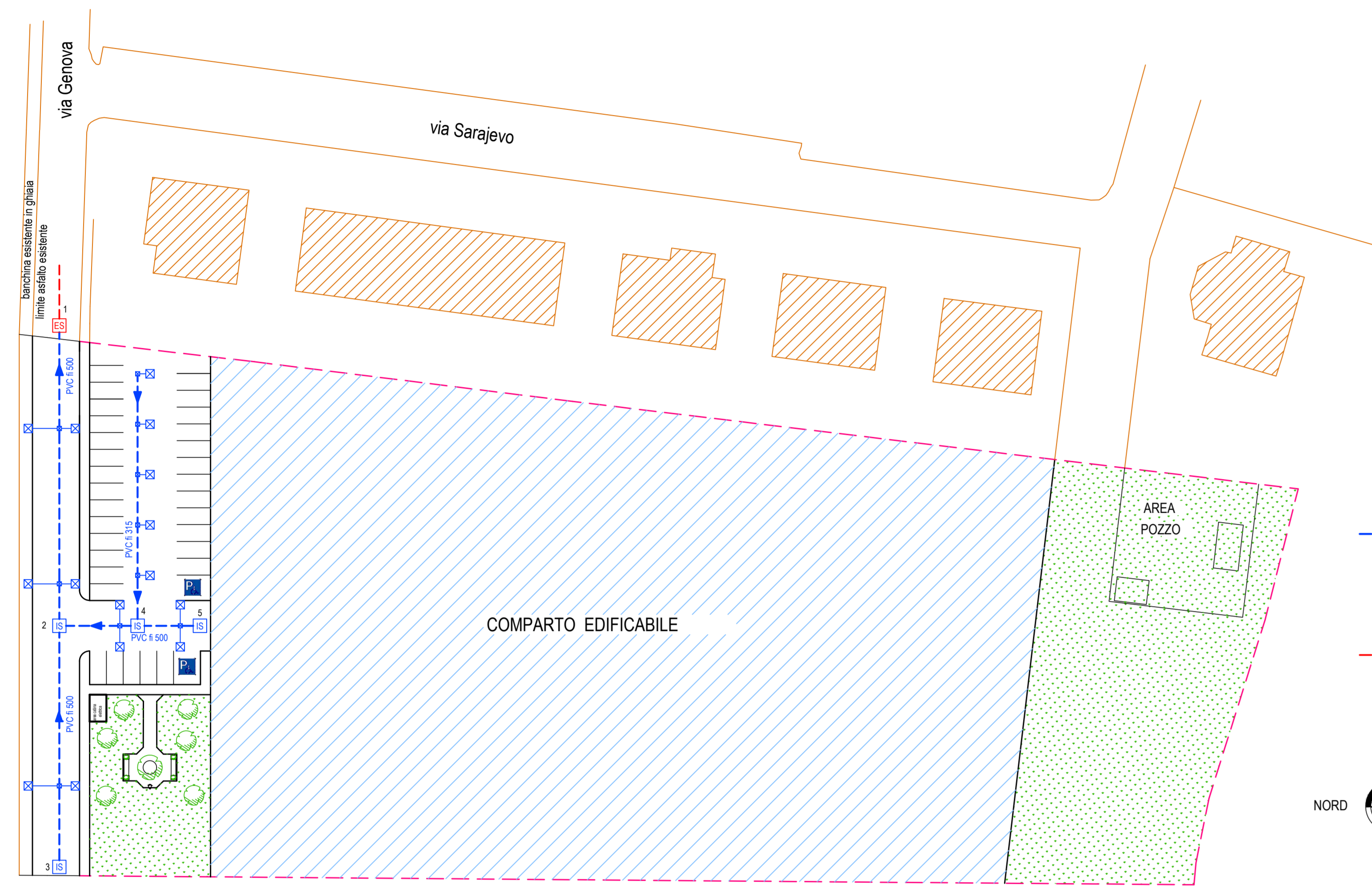
PLANIMETRIA RETE FOGNARIA scala 1:500
